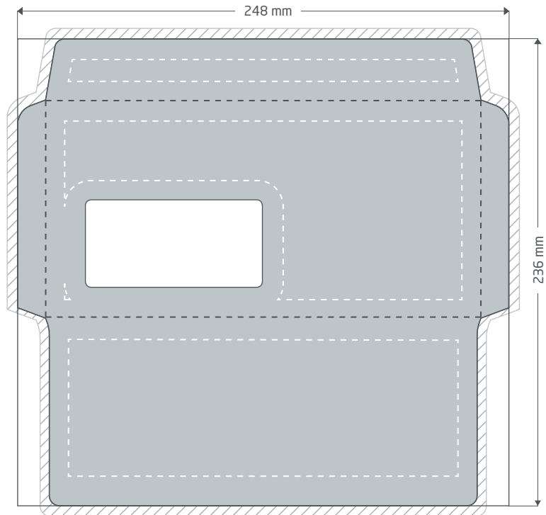
Voorzijde (PDF-pagina 1)
