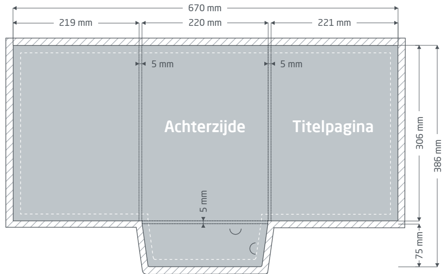
Buitenzijde (PDF-pag. 1)
